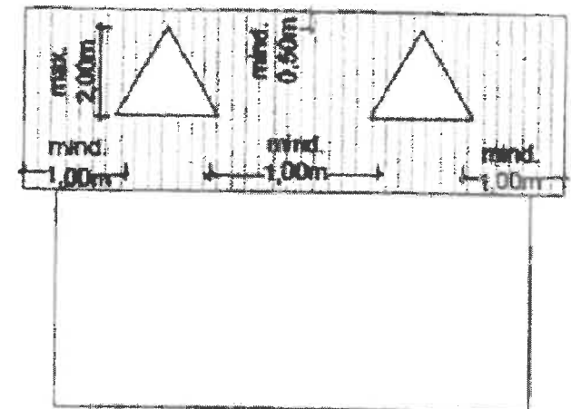
Dreiecksgaube
