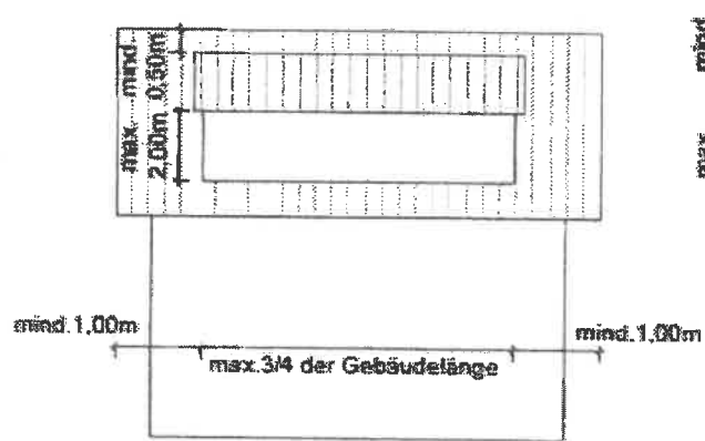
Schleppgaube
